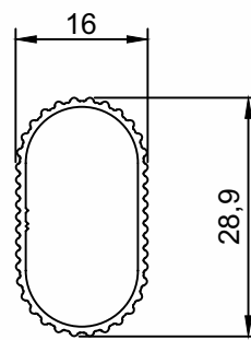
DV-450 Cabideiro Obilongo Peso (Kg/m) Perfis De Encaixe: 0,182
