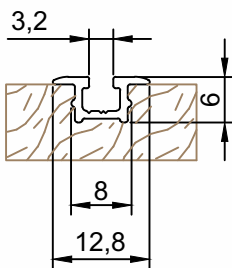
DV-534 Trilho Embutir Peso (Kg/m) Perfis De Encaixe: 0,071
