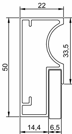
PMO-040 Puxador Porta Peso (Kg/m) Perfis De Encaixe: 0,498
