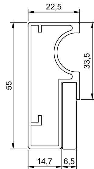
PMO-034 Puxador Porta Peso (Kg/m) Perfis De Encaixe: 0,651
