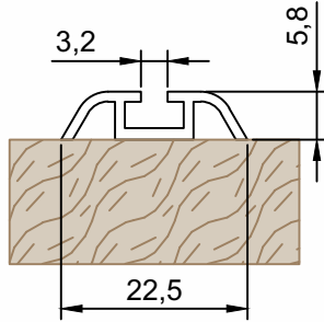
PMO-021 Trilho Inferior Simples Peso (Kg/m) Perfis De Encaixe: 0,133
