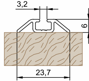
DV-560 Trilho Inferior Simples Peso (Kg/m) Perfis De Encaixe: 0,127
