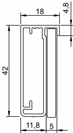
DV-591 Folha Vertical e Horizontal Peso (Kg/m) Perfis De Encaixe: 0,389 DV-593
