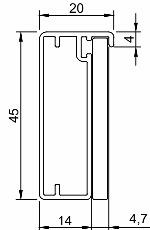
PMO-066 Folha Vertical e Horizontal Peso (Kg/m) Perfis De Encaixe: 0,425 PMO-046
