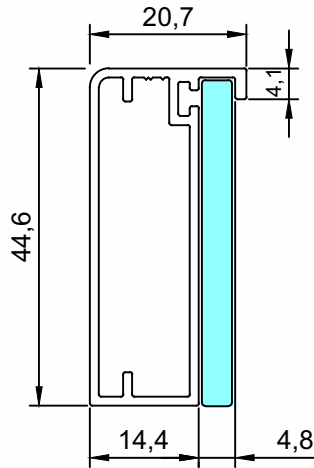
DV-471 Folha Vertical e Horizontal Peso (Kg/m) Perfis De Encaixe: 0,441
