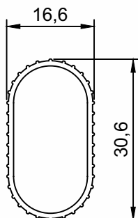
BK-450 Cabideiro Obilongo Peso (Kg/m) Perfis De Encaixe: 0,216
