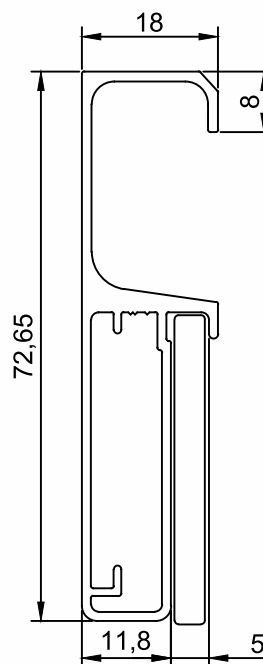
DV-593 Puxador Gola Peso (Kg/m) Perfis De Encaixe: DV-591 0,653
