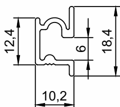
DV-360 Suporte - Caixa De Divisória Peso (Kg/m) Perfis De Encaixe: 0,152
