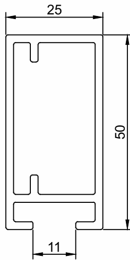
TP-245 Folha Vertical e Horizontal Peso (Kg/m) Perfis De Encaixe: 0,878
