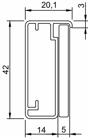
DV-371 Folha Vertical e Horizontal Peso (Kg/m) Perfis De Encaixe: 0,374
