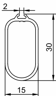
DV-413 Cabideiro Obilongo Peso (Kg/m) Perfis De Encaixe: 0,243
