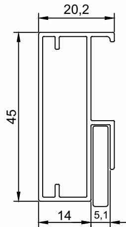
DV-619 Puxador Porta Peso (Kg/m) Perfis De Encaixe: 0,435
