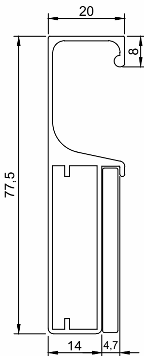
PMO-036 Puxador Gola Peso (Kg/m) 0,733 Perfis De Encaixe: PMO-002
