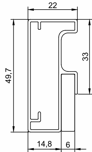
PMO-022 Puxador Porta Peso (Kg/m) Perfis De Encaixe: 0,506
