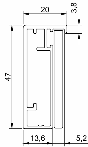
DV-508 Folha Vertical e Horizontal Peso (Kg/m) Perfis De Encaixe: 0,557
