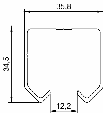
DV-533 Trilho Superior Peso (Kg/m) Perfis De Encaixe: 0,136
