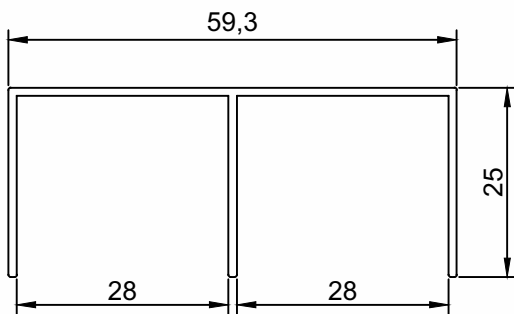
PMO-500 Trilho Superior Peso (Kg/m) Perfis De Encaixe: 0,390 PMO-003 PMO-81
