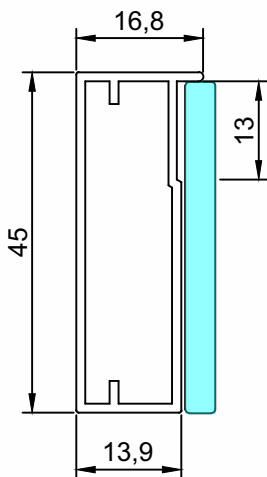
PMO-014 Folha Vertical e Horizontal Peso (Kg/m) Perfis De Encaixe: DV-562 0,393
