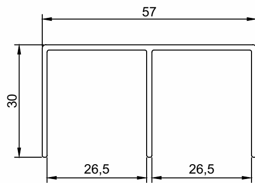
DV-348 Trilho Superior Peso (Kg/m) Perfis De Encaixe: 0,523 PMO-003 PMO-082 DV-638 DV-349
