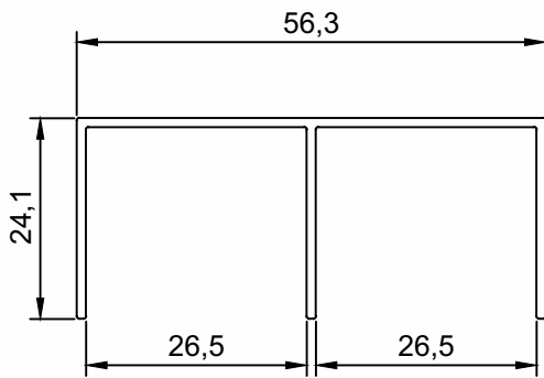
PMO-005 Trilho Superior Peso (Kg/m) Perfis De Encaixe: 0,346 PMO-003 PMO-082 DV-638 DV-349
