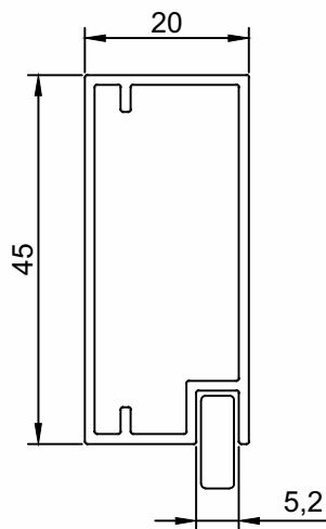
PMO-028 Folha Vertical e Horizontal Peso (Kg/m) Perfis De Encaixe: 0,450
