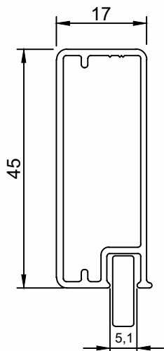
DV-472 Folha Vertical e Horizontal Peso (Kg/m) Perfis De Encaixe: 0,420
