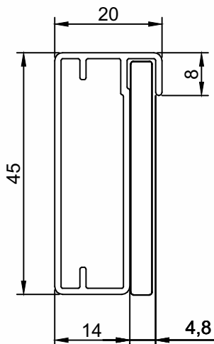
PMO-004 Folha Vertical e Horizontal Peso (Kg/m) Perfis De Encaixe: PMO-016 0,413
