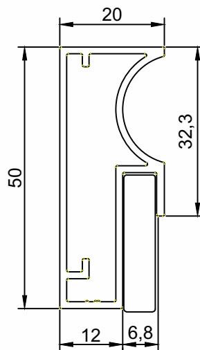
DV-465 Puxador Porta Peso (Kg/m) Perfis De Encaixe: 0,567
