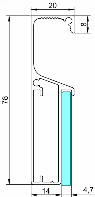
PMO-091 Puxador Gola - Tap Peso (Kg/m) Perfis De Encaixe: PMO-002 0,670
