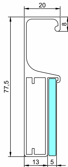
PMO-035 Folha Com Puxador Peso (Kg/m) 0,733 Perfis De Encaixe: PMO-010
