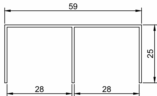
DV-385 Trilho Superior Peso (Kg/m) Perfis De Encaixe: 0,355 PMO-003 PMO-81
