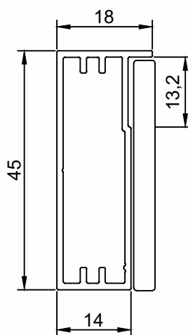
PMO-048 Folha Vertical e Horizontal Peso (Kg/m) Perfis De Encaixe: PMO-020 0,417
