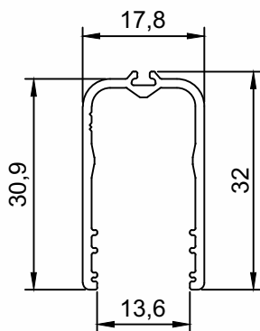
DV-447 Cabideiro Obilongo Peso (Kg/m) Perfis De Encaixe: 0,289
