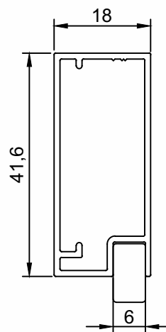
DV-474 Folha Vertical e Horizontal Peso (Kg/m) Perfis De Encaixe: 0,380
