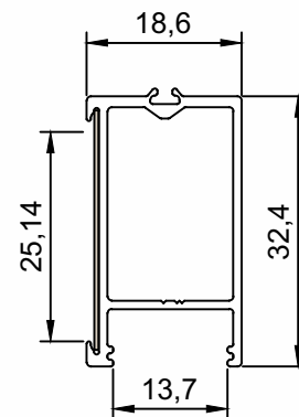
DV-576 Cabideiro C/ Fita De Borda Peso (Kg/m) Perfis De Encaixe: 0,302
