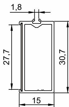
DV-519 Cabideiro C/ Fita De Borda Peso (Kg/m) Perfis De Encaixe: 0,252
