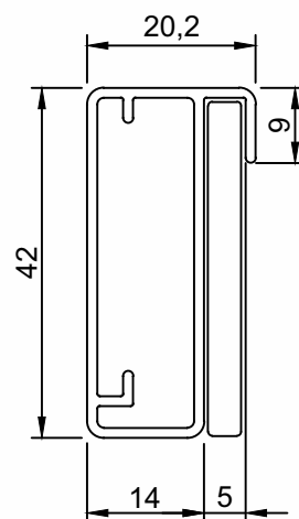
DV-364 Folha Vertical e Horizontal Peso (Kg/m) Perfis De Encaixe: 0,422
