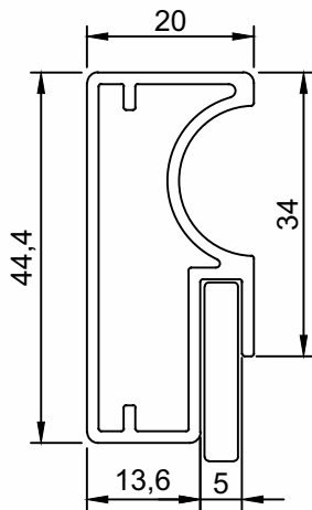
DV-603 Puxador Porta Peso (Kg/m) Perfis De Encaixe: 0,565
