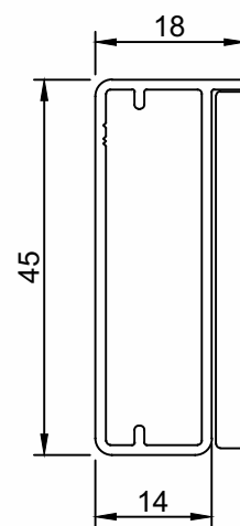
DV-584 Folha Vertical e Horizontal Peso (Kg/m) Perfis De Encaixe: 0,378
